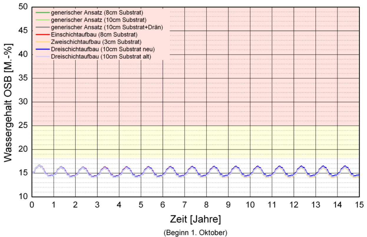
Bild 109: Berechneter Verlauf des Wassergehalts in der OSB-Platte einer Leichtbau- konstruktion mit 20 cm „Isofloc L“, raumseitiger „INTELLO“ und 10 cm Überdämmung der äußeren Schalung in Abhängigkeit von verschiedenen Gründachaufbauten.
