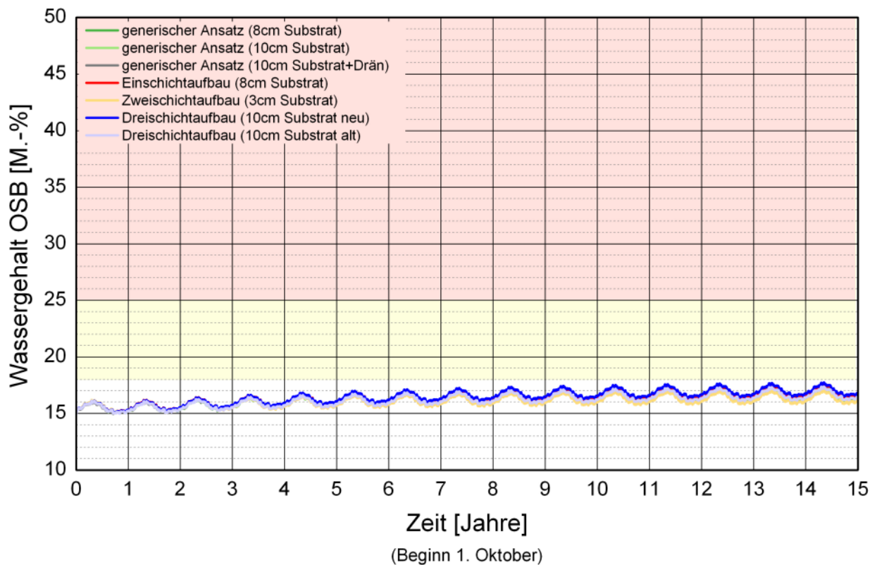
Bild 99: Berechneter Verlauf des Wassergehalts in der OSB-Platte einer Leichtbaukonstruktion mit 40 cm „ISOVER GW Integra ZKF-035“, raumseitiger „Vario Xtra“ und 10 cm Überdämmung der äußeren Schalung in Abhängigkeit von verschiedenen Gründachaufbauten.
