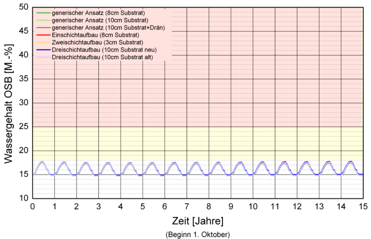
Bild 122: Berechneter Verlauf des Wassergehalts in der OSB-Platte einer Leichtbaukonstruktion mit 40 cm „Isofloc L“, raumseitiger „Vario Xtra“ und 15 cm Überdämmung der äußeren Schalung in Abhängigkeit von verschiedenen Gründachaufbauten.
