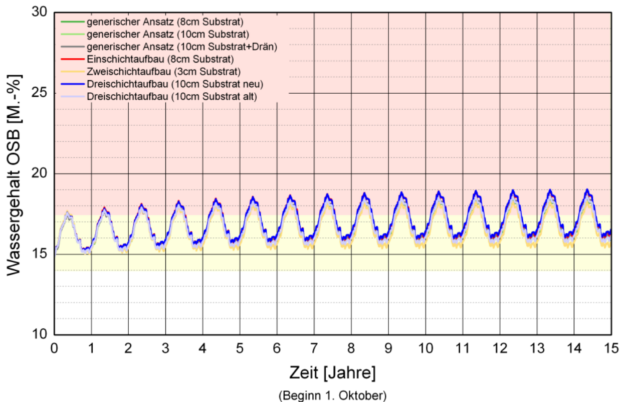
Bild 108: Berechneter Verlauf des Wassergehalts in der OSB-Platte einer Leichtbaukonstruktion mit 20 cm „Isofloc L“, raumseitiger „INTELLO“ und 5 cm Überdämmung der äußeren Schalung in Abhängigkeit von verschiedenen Gründachaufbauten.
