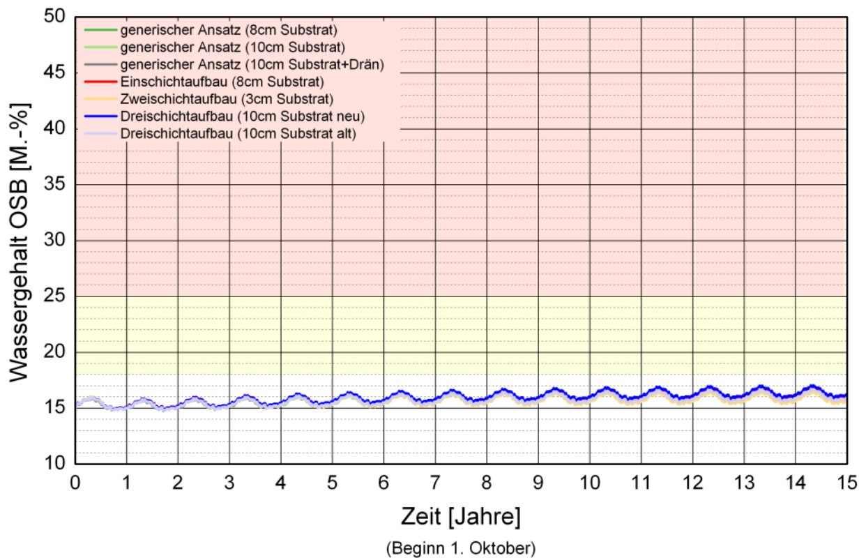
Bild 100: Berechneter Verlauf des Wassergehalts in der OSB-Platte einer Leichtbau- konstruktion mit 40 cm „ISOVER GW Integra ZKF-035“, raumseitiger „Vario Xtra“ und 12 cm Überdämmung der äußeren Schalung in Abhängigkeit von verschiedenen Gründachaufbauten.
