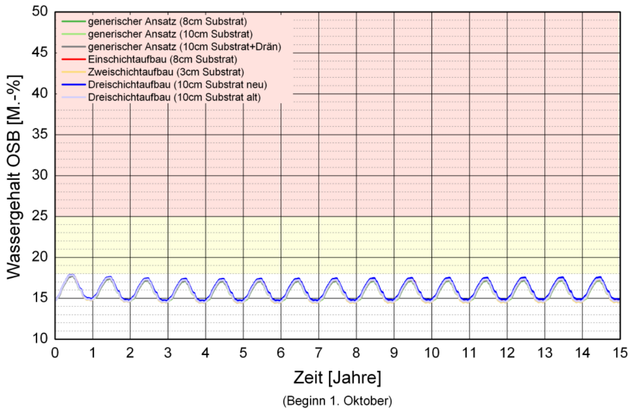
Bild 128: Berechneter Verlauf des Wassergehalts in der OSB-Platte einer Leichtbau- konstruktion mit 40 cm „Isifloc L“, raumseitiger OSB-Platte und 18 cm Überdämmung der äußeren Schalung in Abhängigkeit von verschiedenen Gründachaufbauten.
