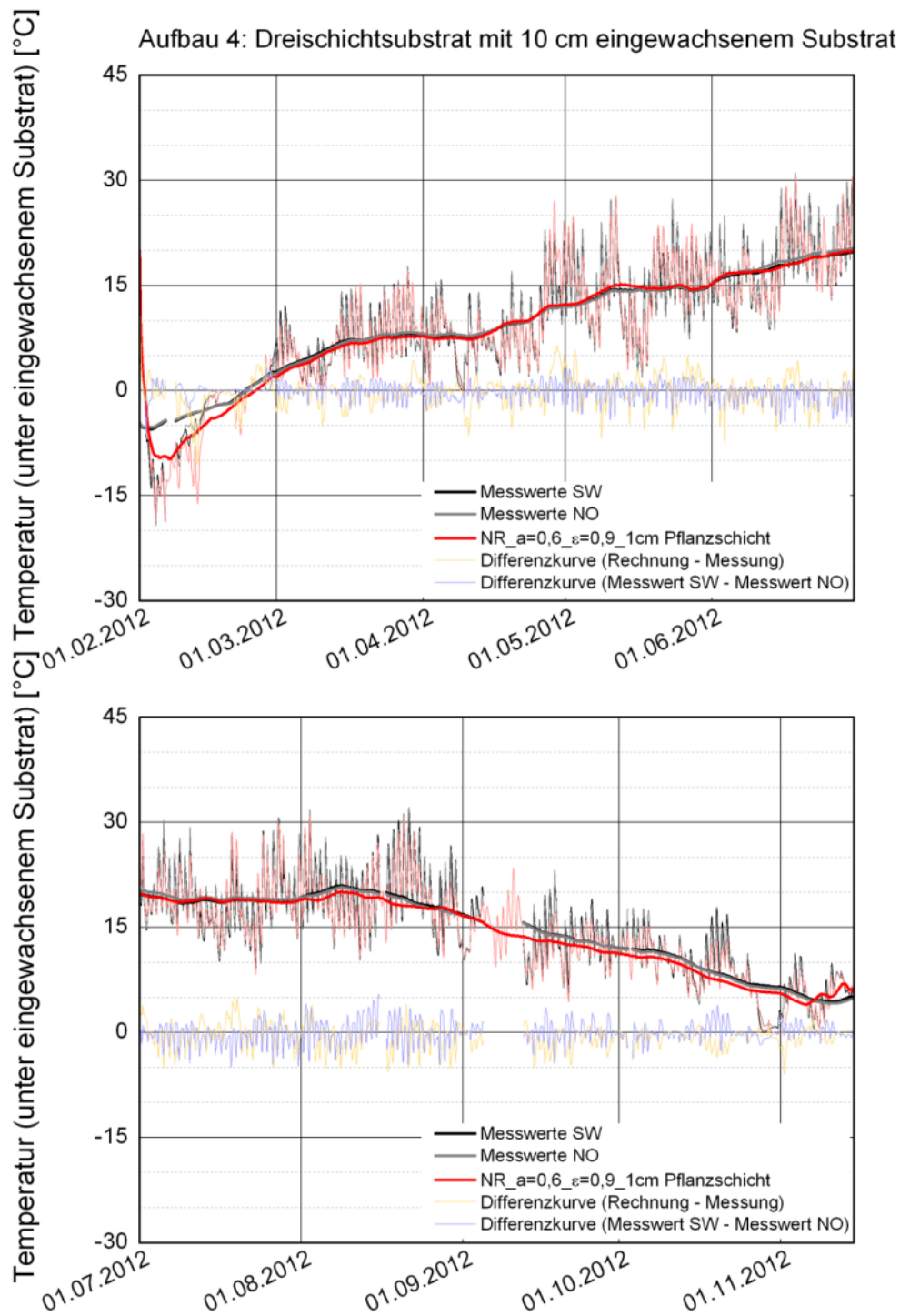
Bild 68: Berechneter Verlauf der Temperaturen unter dem eingewachsenen Substrat von Dachaufbau 4 mit einer 1cm dicken Pflanzschicht (rot) im Vergleich zu den beiden Messkurven (grau / schwarz). Die hellen Kurven stellen die stündlichen Werte dar, die dunklen Kurven das gleitende Monatsmittel.
