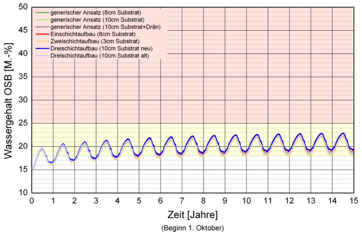
Bild 124: Berechneter Verlauf des Wassergehalts in der OSB-Platte einer Leichtbaukonstruktion mit 40 cm „Isfloc L“, raumseitiger OSB-Platte und 5 cm Überdämmung der äußeren Schalung in Abhängigkeit von verschiedenen Gründachaufbauten.
