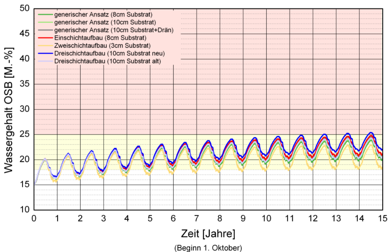
Bild 110: Berechneter Verlauf des Wassergehalts in der OSB-Platte einer Leichtbaukonstruktion mit 40 cm „Isfloc L“ und raumseitiger „INTELLO“ ohne Überdämmung der äußeren Schalung in Abhängigkeit von verschiedenen Gründachaufbauten.
