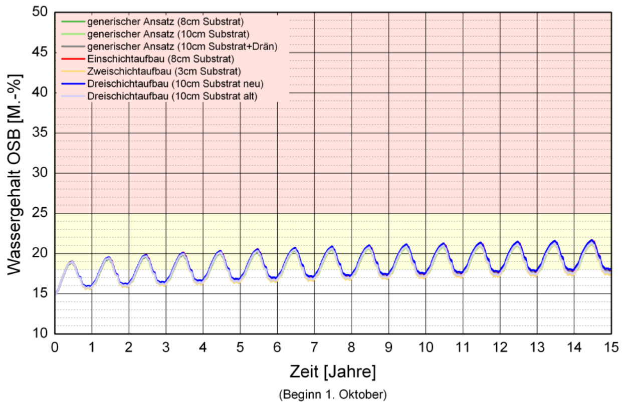
Bild 119: Berechneter Verlauf des Wassergehalts in der OSB-Platte einer Leichtbaukonstruktion mit 40 cm „Isofloc L“, raumseitiger „Vario Xtra“ und 5 cm Überdämmung der äußeren Schalung in Abhängigkeit von verschiedenen Gründachaufbauten.
