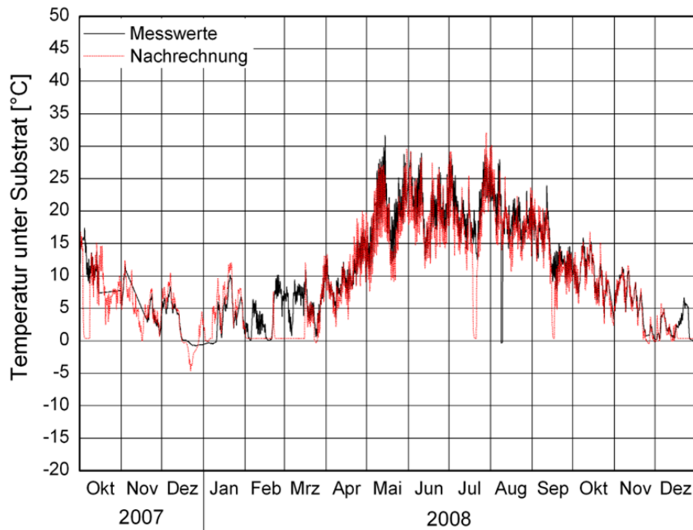
Bild 28: Berechneter Verlauf der Temperatur unter der Substratschicht des Gründachversuchsfeldes „Feld II“ am Standort Kassel im Vergleich zu den gemessenen Werten für den Messzeitraum Oktober 2007 bis Dezember 2008.
