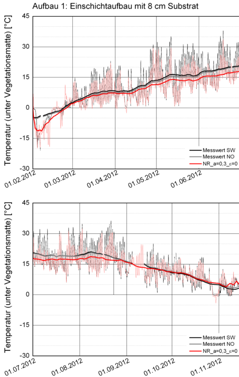
Bild 57: Berechneter Verlauf der Temperaturen unter der Vegetationsmatte von Dachaufbau 1 mit dem generischen Berechnungsmodell (rot) im Vergleich zu den beiden Messkurven (grau / schwarz). Die hellen Kurven stellen die stündlichen Werte dar, die dunklen Kurven das gleitende Monatsmittel.
