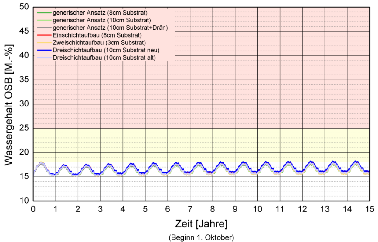
Bild 105: Berechneter Verlauf des Wassergehalts in der OSB-Platte einer Leichtbau- konstruktion mit 40 cm „ISOVER GW Integra ZKF-035“, raumseitiger OSB- Platte und 15 cm Überdämmung der äußeren Schalung in Abhängigkeit von verschiedenen Gründachaufbauten.
