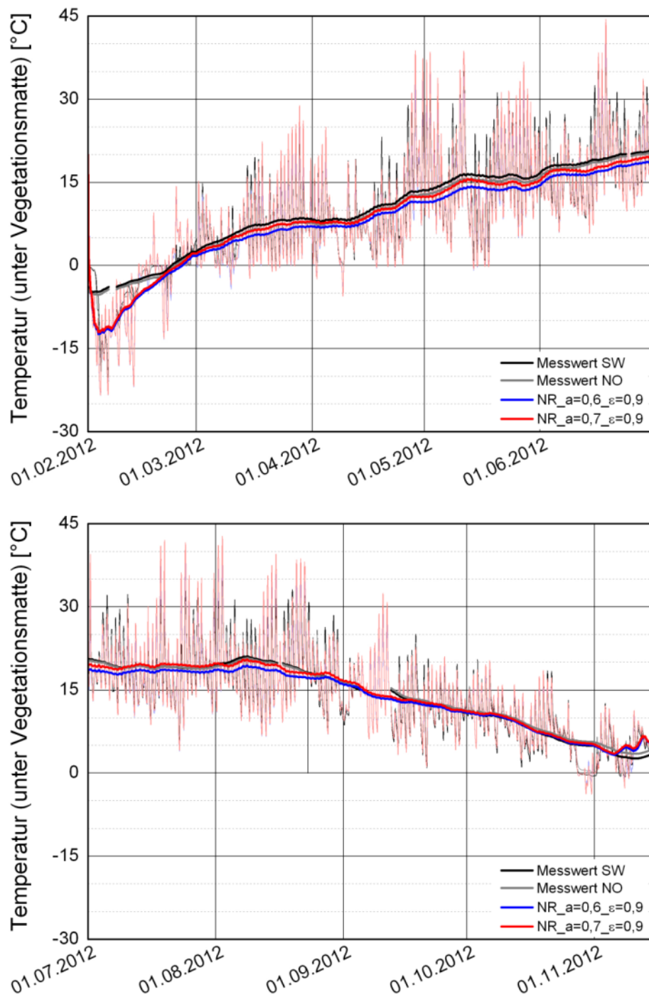
Aufbau 1: Einschichtaufbau mit 8 cm Substrat
