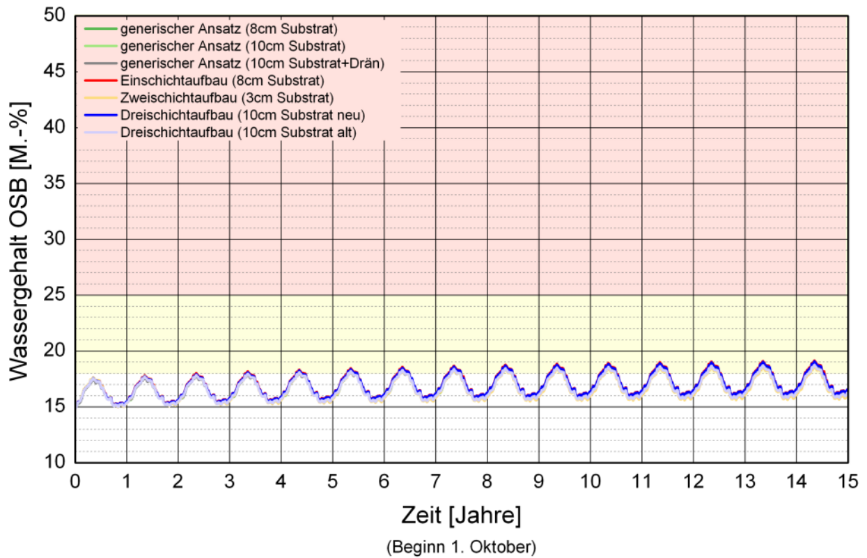
Bild 116: Berechneter Verlauf des Wassergehalts in der OSB-Platte einer Leichtbaukonstruktion mit 20 cm „Isofloc L“, raumseitiger „Vario Xtra“ und 5 cm Überdämmung der äußeren Schalung in Abhängigkeit von verschiedenen Gründachaufbauten.
