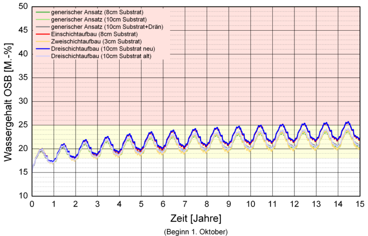
Bild 102: Berechneter Verlauf des Wassergehalts in der OSB-Platte einer Leichtbau- konstruktion mit 40 cm „ISOVER GW Integra ZKF-035“, raumseitiger OSB- Platte und 5 cm Überdämmung der äußeren Schalung in Abhängigkeit von verschiedenen Gründachaufbauten.
