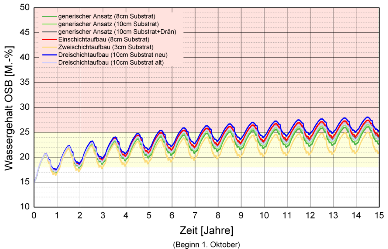
Bild 123: Berechneter Verlauf des Wassergehalts in der OSB-Platte einer Leichtbau- konstruktion mit 40 cm „Isofloc L“ und raumseitiger OSB-Platte ohne Überdämmung der äußeren Schalung in Abhängigkeit von verschiedenen Gründachaufbauten.
