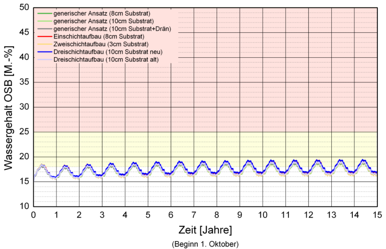
Bild 104: Berechneter Verlauf des Wassergehalts in der OSB-Platte einer Leichtbau- konstruktion mit 40 cm „ISOVER GW Integra ZKF-035“, raumseitiger OSB- Platte und 12 cm Überdämmung der äußeren Schalung in Abhängigkeit von verschiedenen Gründachaufbauten.
