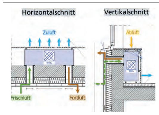
Abb. 75 Luftein- und -auslässe des DFL-Gerätes (TROX 10/2016)
