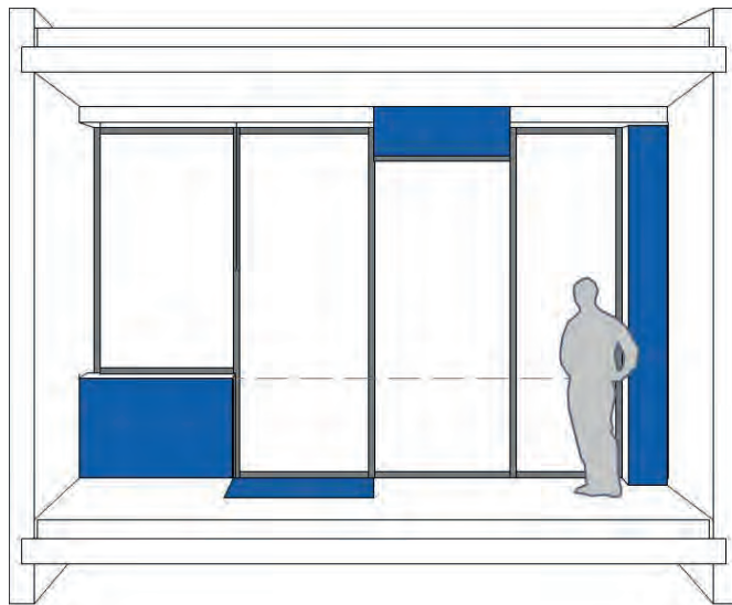
Abb. 7 Einbausituationen für DFL-Geräte mit Bezug zur vertikalen Zonierung von Fassaden (THN-AR)
