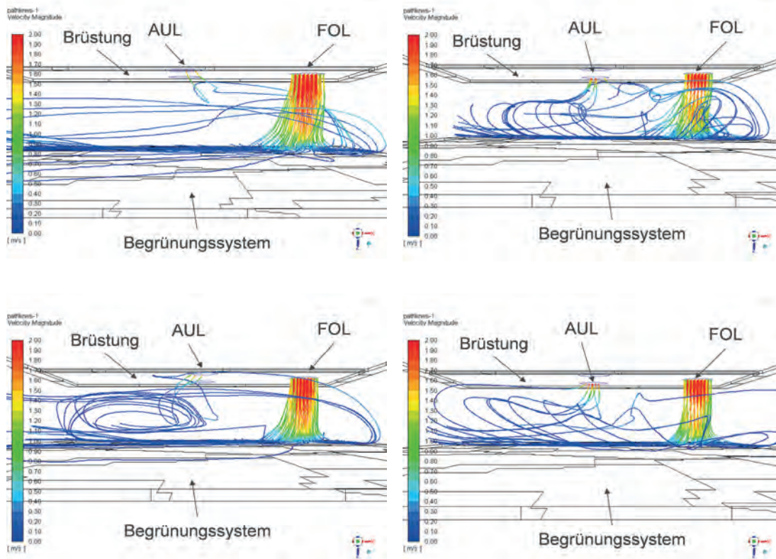
Abb. 32 – 35 Draufsicht des Spalts zwischen Fassade und den wandgebundenen Begrünungssystemen Vertiko und Verticalgreendesign (VGD) mit der Außenluftansaugung (AUL) und Fortluftausbringung (FOL). Es sind die Strömungslinien der Luftpartikel, eingefärbt nach ihrer Geschwindigkeit, ausgehend von der Fortluftausbringung für beide Systeme jeweils für die Ansaugung im oberen und unteren Brüstungsbereich, dargestellt. Als Strömungslinien werden Strömungswege bezeichnet, die die Fluidteilchen beim Strömen nehmen.
