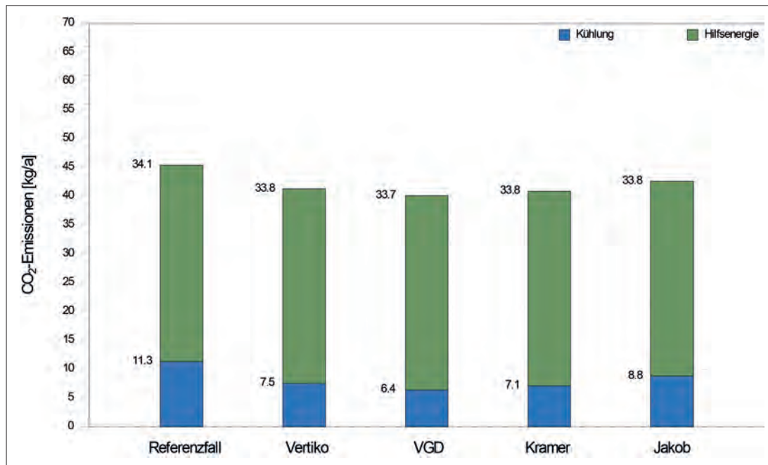
Abb. 64 CO 2 -Emissionen des Fassadenlüftungssystems. Referenzfall und in Kombination mit den untersuchten Begrünungssysteme – Ergebnisse Simulation Fassadenversuchsstand Rednitzhembach (THN-ieg)
