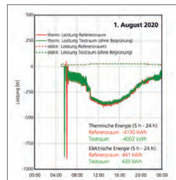
Abb. A60 Thermische (wasserseitig) und elektrische Leistung der DFL in den Zwillingräumen am 1. August 2020 (IBP)
