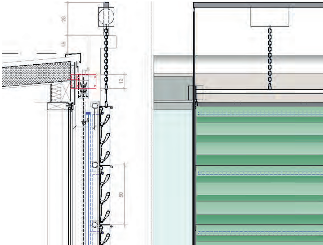
Abb. A3 Rednitzhembach, Technikum/ Fassadenversuchsstand – Traufdetail (o. M.) (THN-AR)
