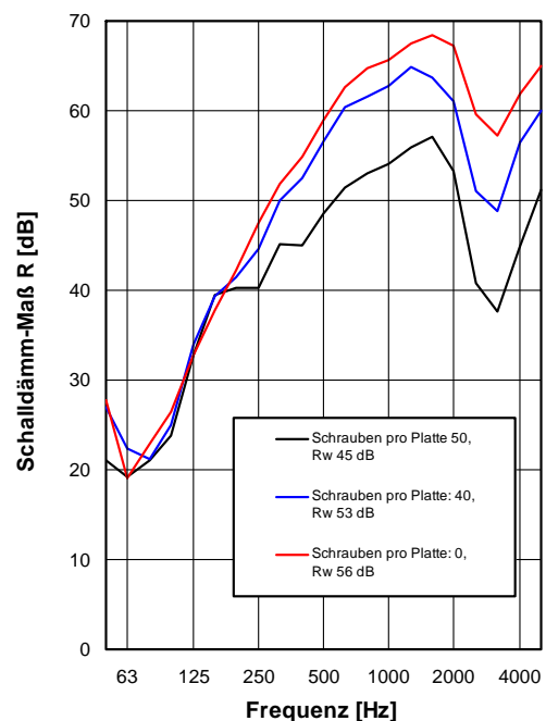
Bild 9: Schalldämmung von Wandausschnitten im Fensterprüfstand bei unterschiedlicher Schraubenanzahl.
