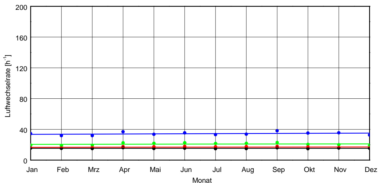
Bild 41: Berechneter, monatlicher Luftwechsel in der Doppelfassade bei Veränderung des äußeren Verglasungstyps.
