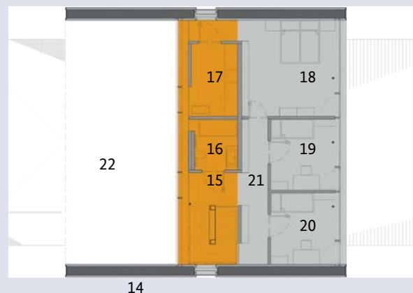
Grundriss Obergeschoss Wohnnutzung
