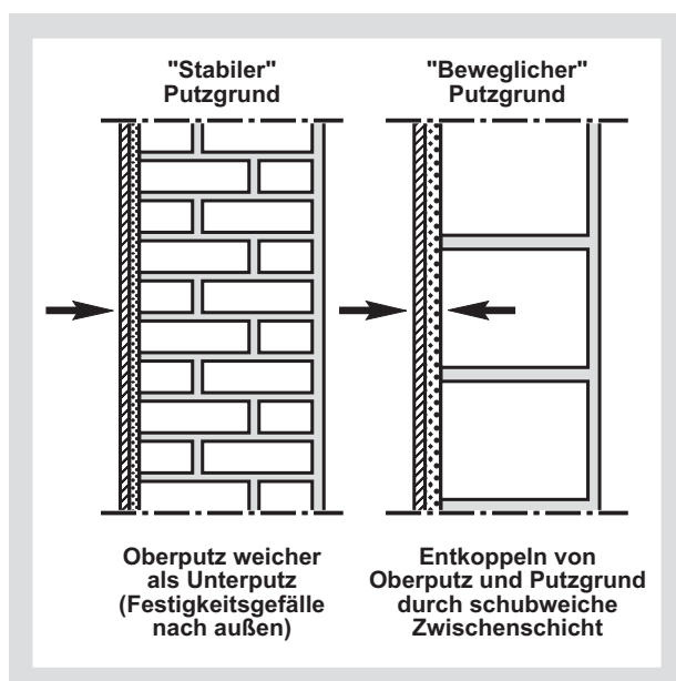
Bild 1: Zuordnung von Putzgrund und Putzsystem. Bei "stabilem" Putzgrund gilt die Putzregel "weich auf hart". Hier sind nur die Klimaeinwirkungen von außen (Pfeil) zu berücksichtigen. Bei "beweglichem" Putzgrund gilt die Putzregel "Entkoppeln", um Einwirkungen von außen und vom Putzgrund her zu begegnen (Pfeile).
