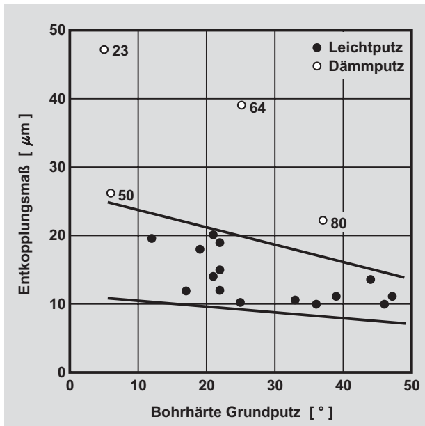
Bild 3: Meßergebnisse des Entkopplungsmaßes von handelsüblichen Putzsystemen, bestehend aus 15 mm Grundputz und 5 mm Deckputz, in Abhängigkeit von der Bohrhardt des Grundputzes. Die Zahlen bei den Meßwerten der Putzsysteme mit Wärmedämm-Grundputz bedeuten die Bohrhardt der Deckputze. Bei den Leicht-Grundputzen liegen die Bohrhardtewerte der Deckputze mehrheitlich (80 %) im Bereich zwischen 45 und 70°. Sowohl bei Leichtputzen als auch bei Dämmputzen ist eine abnehmende Tendenz des Entkopplungsmaßes mit zunehmender Härte des Grundputzes festzustellen.
