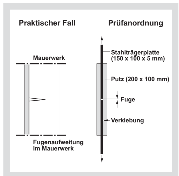
Bild 2: Schemadarstellung der Rißursache in der Praxis infolge Fugenaufweitung im Mauerwerk und der Prüfanordnung "Schervogel" zur Ermittlung des Entkopplungsmasses. Aus Symmetriegründen werden gleiche Putzproben beidseitig auf den Stahlträgerplatten aufgeklebt.
