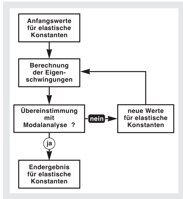
Bild 2: Iterative Bestimmung der elastischen Konstanten
