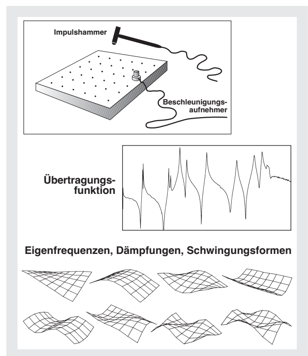
Bild 1: Ermittlung von Eigenschwingungen durch Modalanalyse
