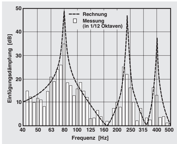
Bild 3: Vergleich der gemessenen und berechneten Dämpfungswerte eines 2 m langen Schalldämpfers (links in Bild 2 dargestellt).
