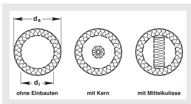
Bild 1: Querschnitte von Rohrschalldämpfern ohne und mit Einbauten.
