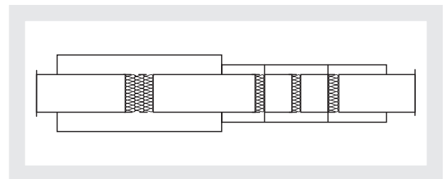
Bild 2: Längsschnitt durch einen 4 m langen Rohr-Schalldämpfer mit 400 mm Durchmesser des Innen-Rohres.
