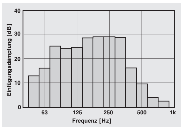
Bild 4: Dämpfungswerte des in Bild 2 dargestellten Rohr-Schalldämpfers in Abhängigkeit von den Terzbändern.
