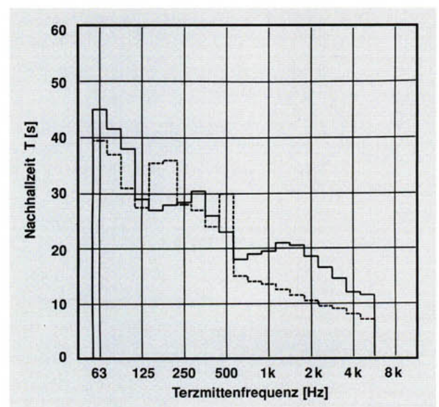
Bild 2: Nachhallzeit T des Kellergewölbes nach Bild 1
