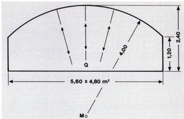
Bild 3: Schematische Darstellung der Schall-Konzentration in dem Gewölbe mit kreisförmiger Begrenzungsfläche M: Kreis-Mittelpunkt; Q: Schallquelle
