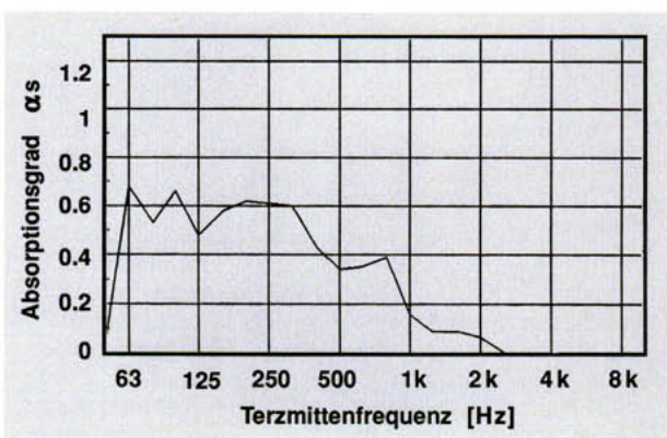
Bild 4: Absorptionsgrad \alpha_s von 10 cm dicken Membran-Absorber-Kassetten, die auf den speziellen Bedarf im Kellergewölbe der Musikschule abgestimmt wurden
