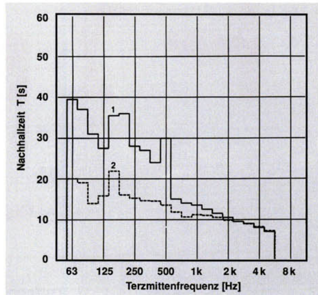
Bild 5: Nachhallzeit T des Musikraumes mit Instrumenten 1 ohne Membran-Absorber-Kassetten 2 mit zehn Membran-Absorber-Kassetten à 0,45 m 2 (gemäß Bild 4)
